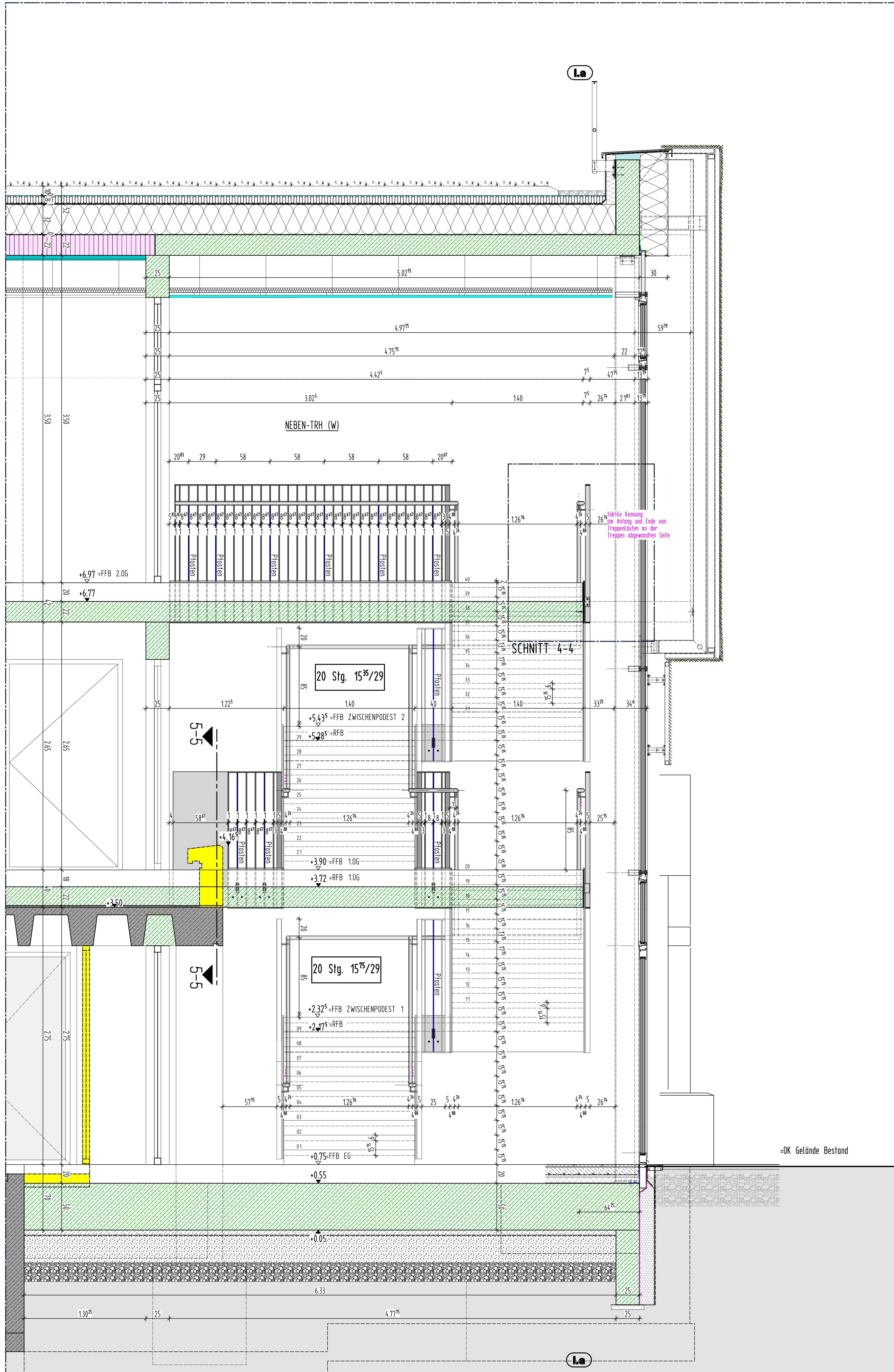
SNITT BB-BB M 1:20
